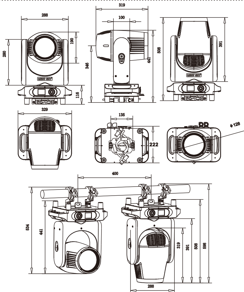
Size-Fig.2 (Unit:mm)
